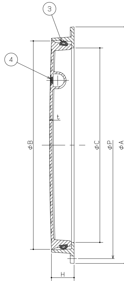
X-0-Y断面
