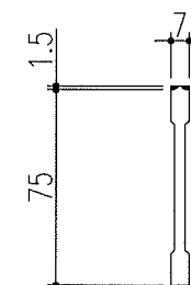
ベアリングバー 詳細図
