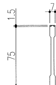
ベアリングバー 詳細図
