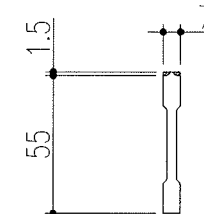
ベアリングバー 詳細図
