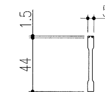
ベアリングバー 詳細図
