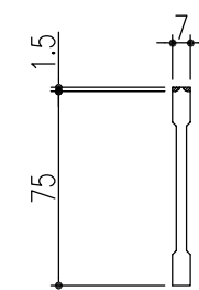
ベアリングバー 詳細図
