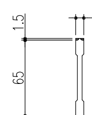
ベアリングバー 詳細図
