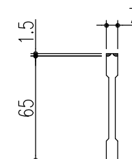
ベアリングバー 詳細図
