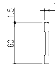
ベアリングバー 詳細図
