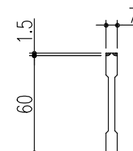
ベアリングバー 詳細図
