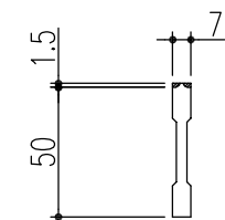
ベアリングバー 詳細図
