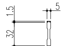
ベアリングバー 詳細図
