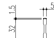
ベアリングバー 詳細図
