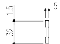
ベアリングバー 詳細図
