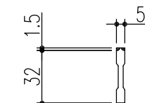
ベアリングバー 詳細図
