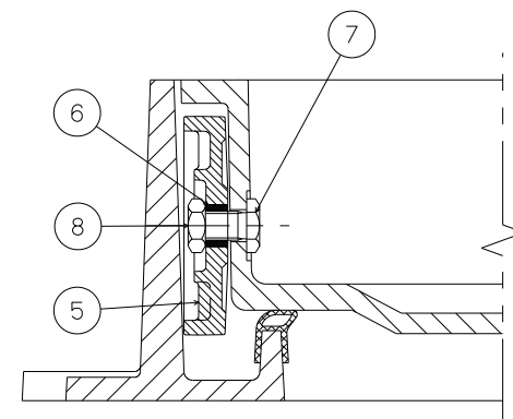
断面Z-Z
