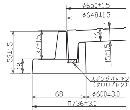
蓋・受枠断面詳細図
