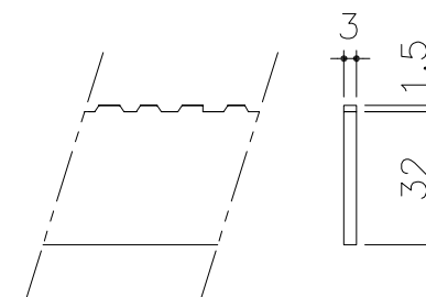
ベアリングバー詳細図
