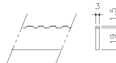
ベアリングバー詳細図
