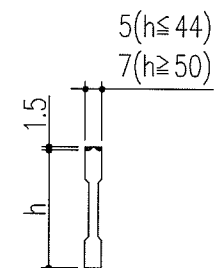
ベアリングバー 詳細図
