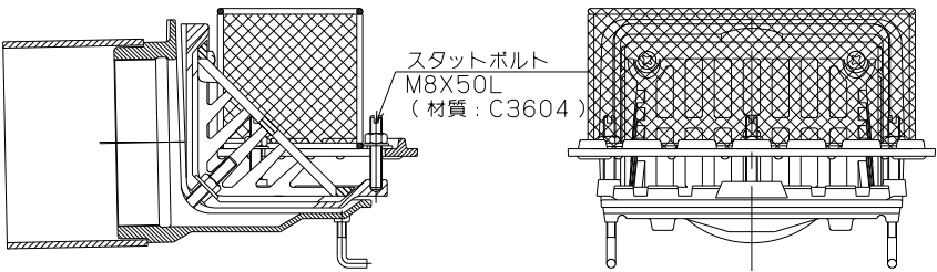
組図
