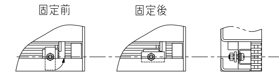
グレーチング固定部詳細図
