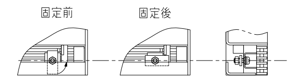
グレーチング固定部詳細図
