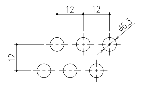
底面排水穴形状 S=1/1
