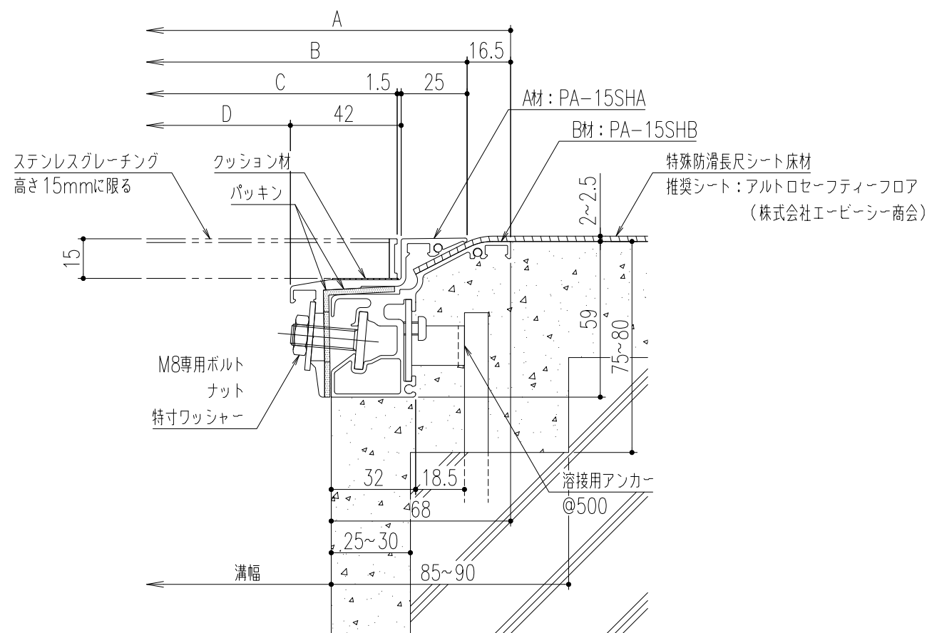
断面詳細図
