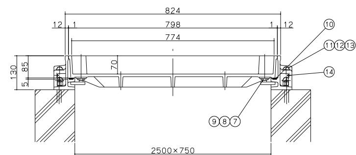
断面図 S=1/5
