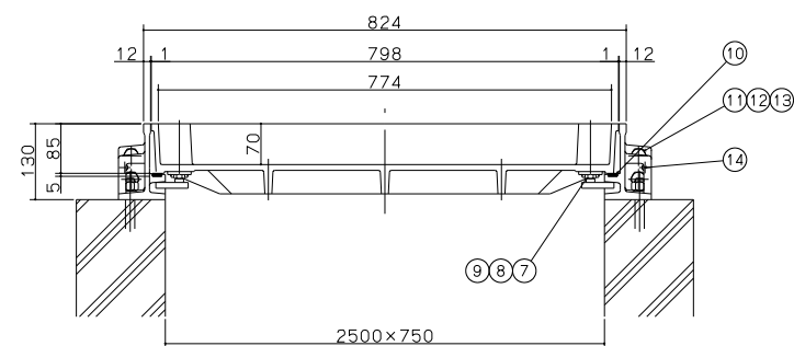
断面図 S=1/5
