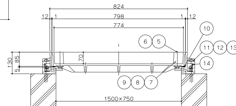
断面図 S=1/5
