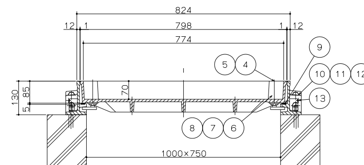
断面図 S=1/5
