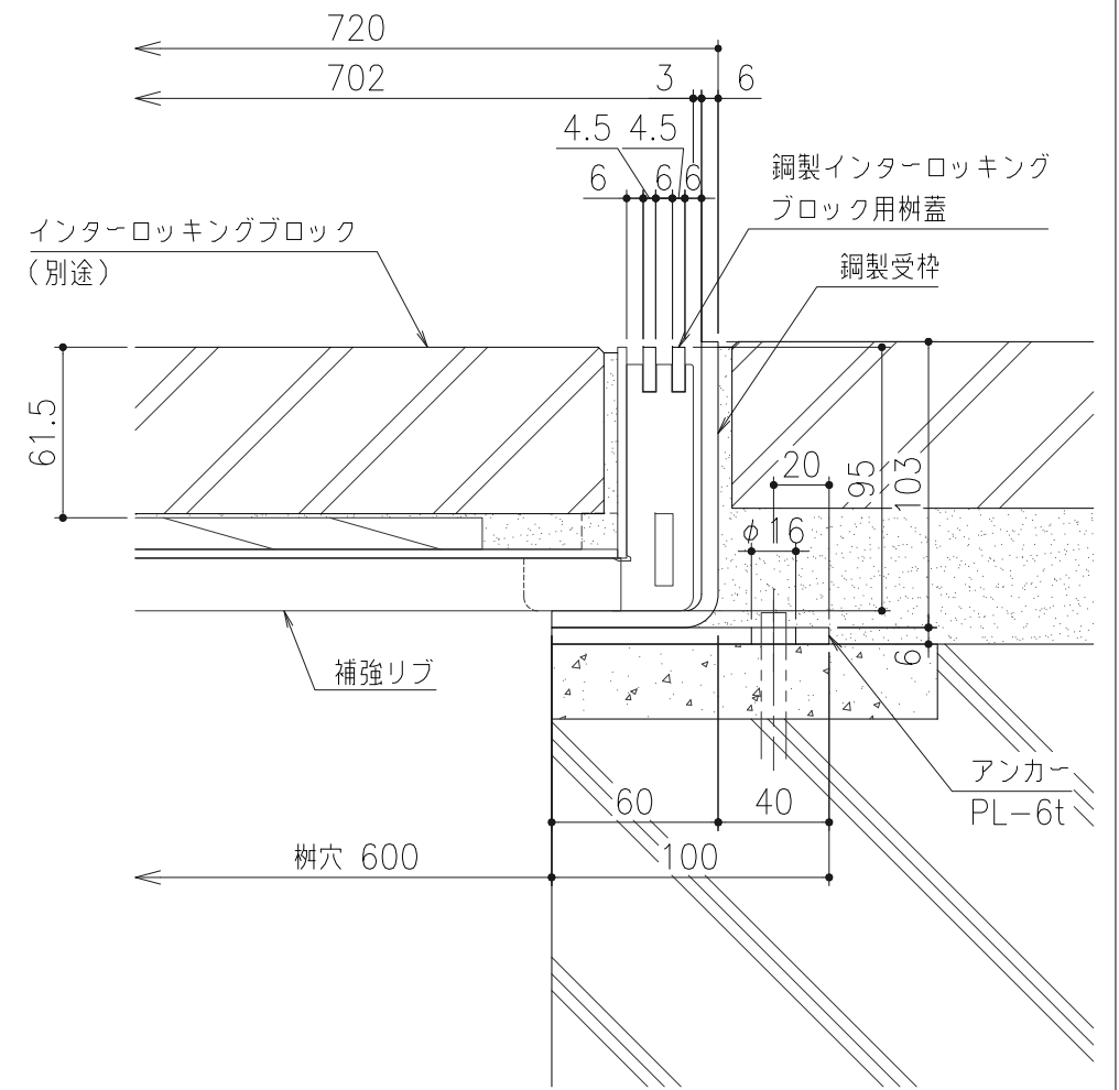
断面詳細図 S=1/3
