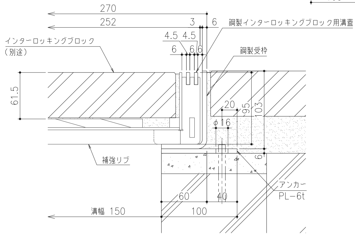
断面詳細図 S=1/3
