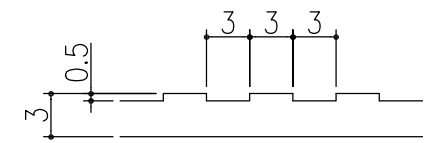
先端カバー 断面詳細図
