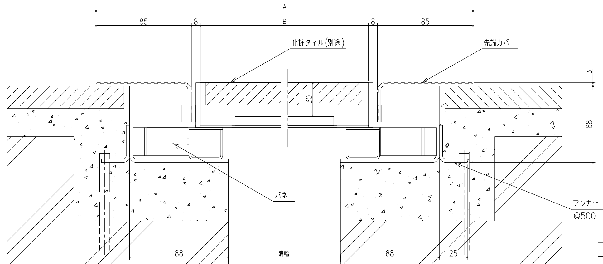
断面詳細図 S=1/2
