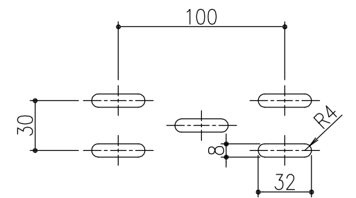
先端カバー 排水穴形状
