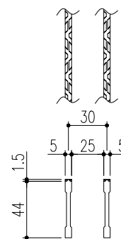
ベアリングバー 詳細図
