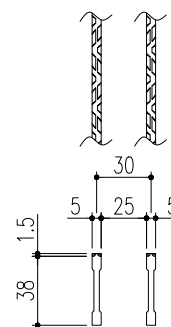
ベアリングバー 詳細図
