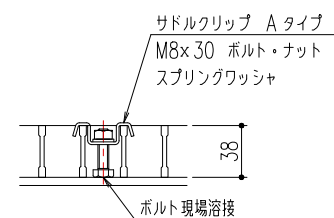
サドルクリップ Aタイプ固定 1/4
