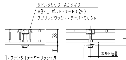
サドルクリップ ACタイプ固定 1/4
