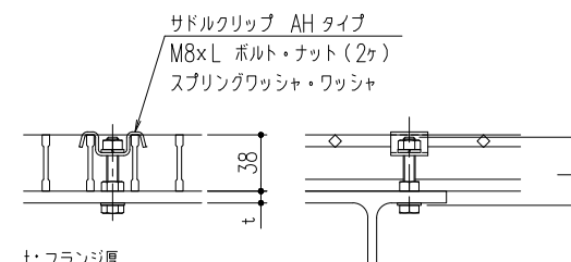
サドルクリップ AHタイプ固定 1/4
