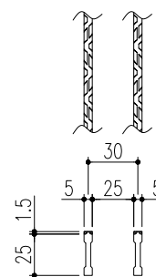
ベアリングバー 詳細図
