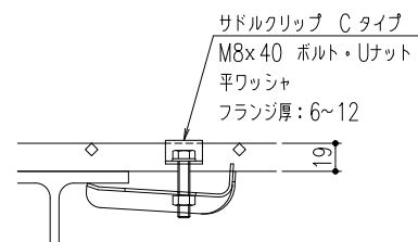
サドルクリップ Cタイプ固定 1/4
