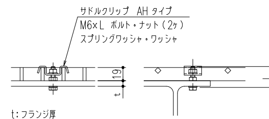
サドルクリップ AHタイプ固定 1/4
