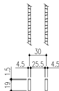
ベアリングバー 詳細図
