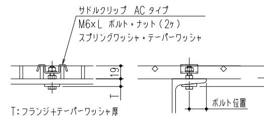
サドルクリップ ACタイプ固定 1/4
