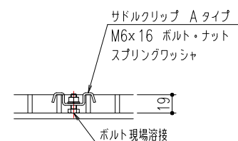
サドルクリップ Aタイプ固定 1/4
