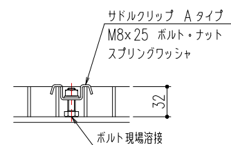
サドルクリップ Aタイプ固定 1/4
