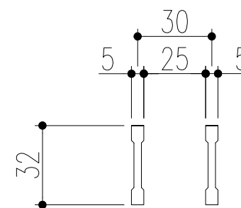
ベアリングバー 詳細図
