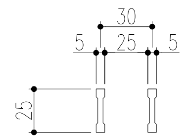
ベアリングバー 詳細図
