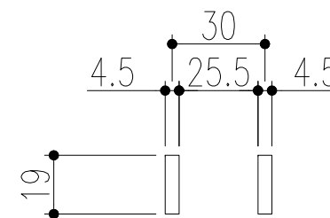
ベアリングバー 詳細図
