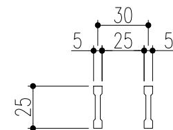
ベアリングバー 詳細図
