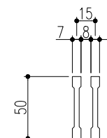
ベアリングバー 詳細図
