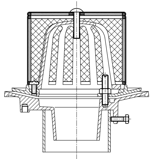
組図 S=1/3
