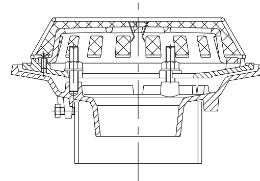
組図
