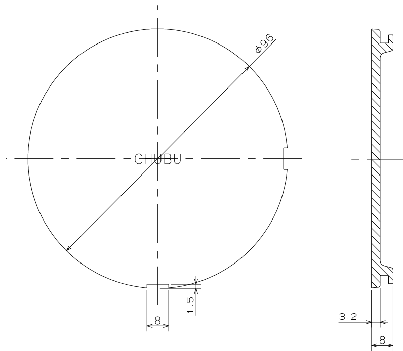
化粧蓋 ( 3-50F )
