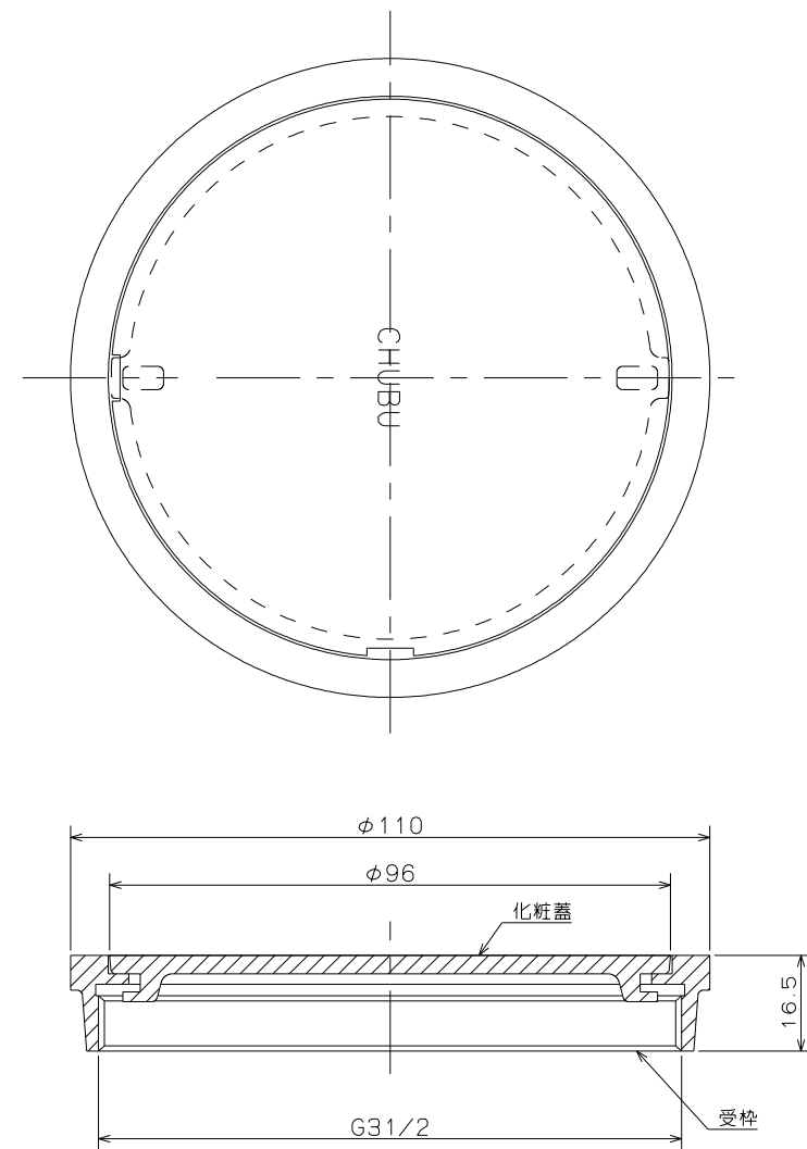
蓋組立て図
