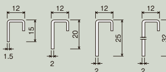
■ベアリングバー断面図
