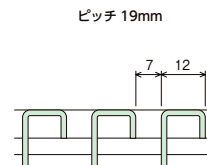
■ベアリングバーピッチ
