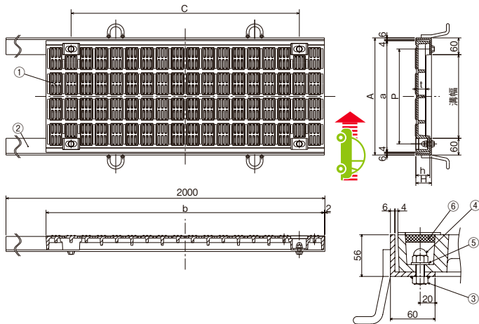
固定部詳細
