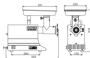
寸法(mm)
